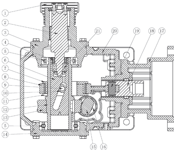
Рис. 3 Приводная часть гидромеханического насоса серии JYP
