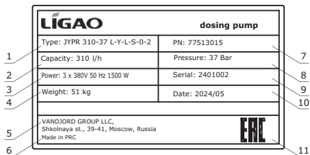
Рис. 2 Фирменная табличка JYPR
