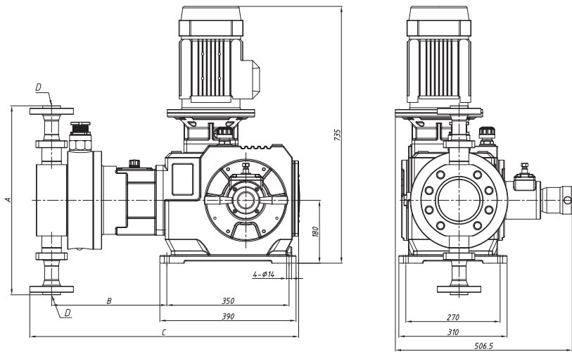
Рис. 24 Габаритные размеры YYPD
